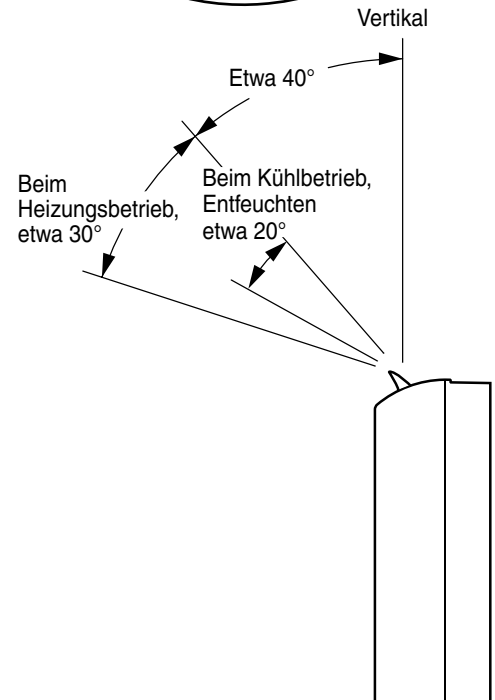
Vertikaler Luftflügel
